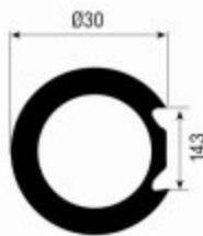
AKM 02.1 30x1.8 mm. 680 gr/m
