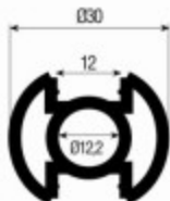
AKM 02.1 30x1.8 mm. 680 gr/m
