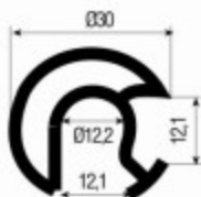
AKM 02 30x1.8 mm. 620 gr/m
