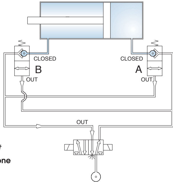
Cilindro Bloccato Stopped Cylinder
